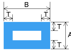
角パイプ(材質 A6063)
