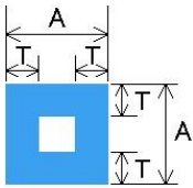
四角パイプ(材質 A6063)
